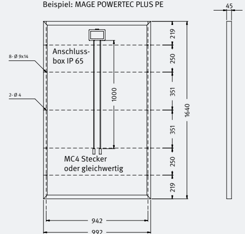
Modullängen: PH 1636, PO 1650, PJ/PR 1655 Zeichnungen auf Anfrage. Alle Längenangaben in mm.
